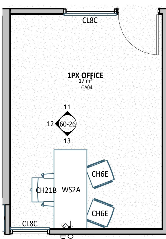
10 PLAN DETAIL 1 : 50
