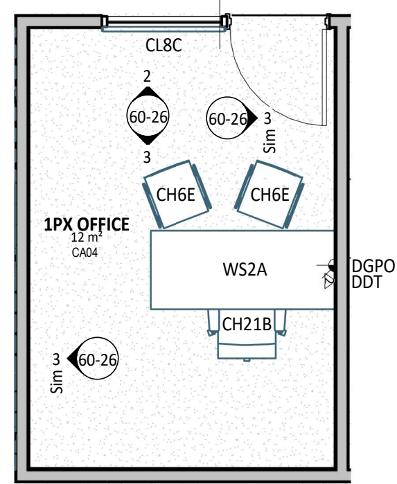
1 PLAN DETAIL 1 : 50
